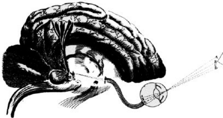
Σχεδιάγραμμα του Καρτέσιου, όπου φαίνονται οι ιδέες του σχετικά με το πώς ο εγκέφαλος σχηματίζει νοητικές εικόνες ενός αντικειμένου. Η αλληλεπίδραση νοητικής ουσίας και σωματικής ουσίας υποτίθεται ότι γίνεται στην επίφυση (H).
